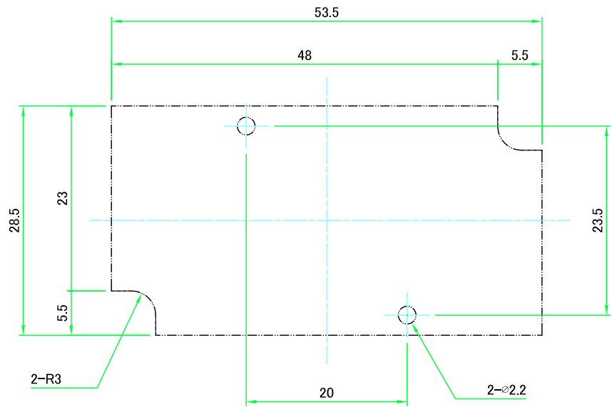
推奨基板形状 * 販売していません Recommended PCB dimension * NOT SUPPLIED
